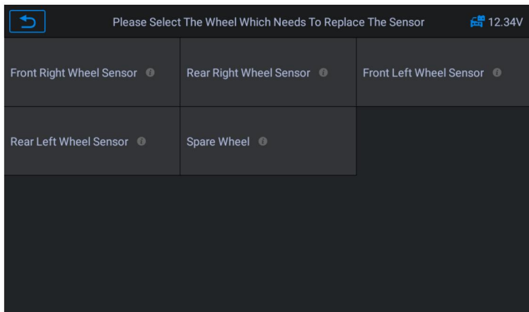
Obrázek 5-58 Ukázková obrazovka funkce TPMS 3
