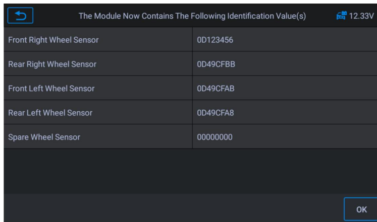
Obrázek 5-63 Ukázková obrazovka funkce TPMS 8
