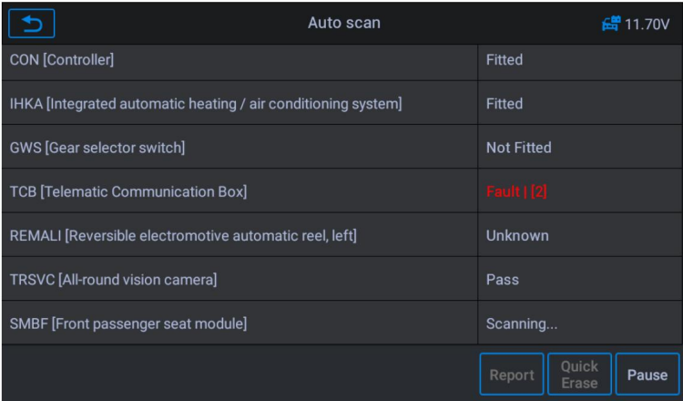
Obrázek 4-13 Ukázka obrazovky automatického skenování
