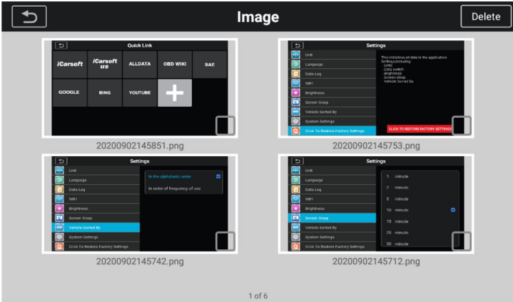
Obrázek 6-2 Ukázková obrazovka
